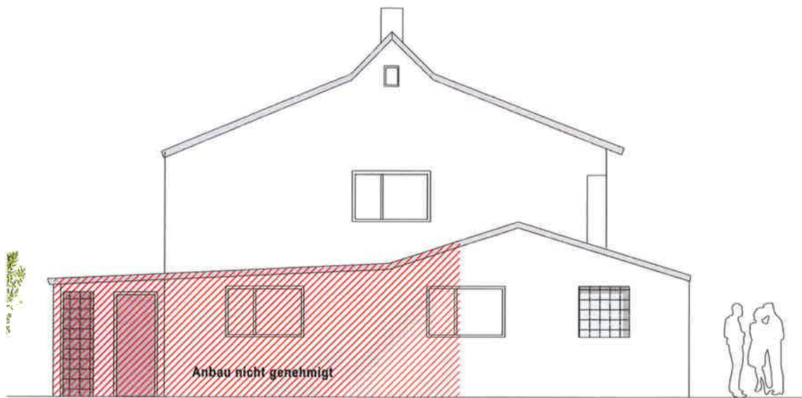
Ansicht Ost
