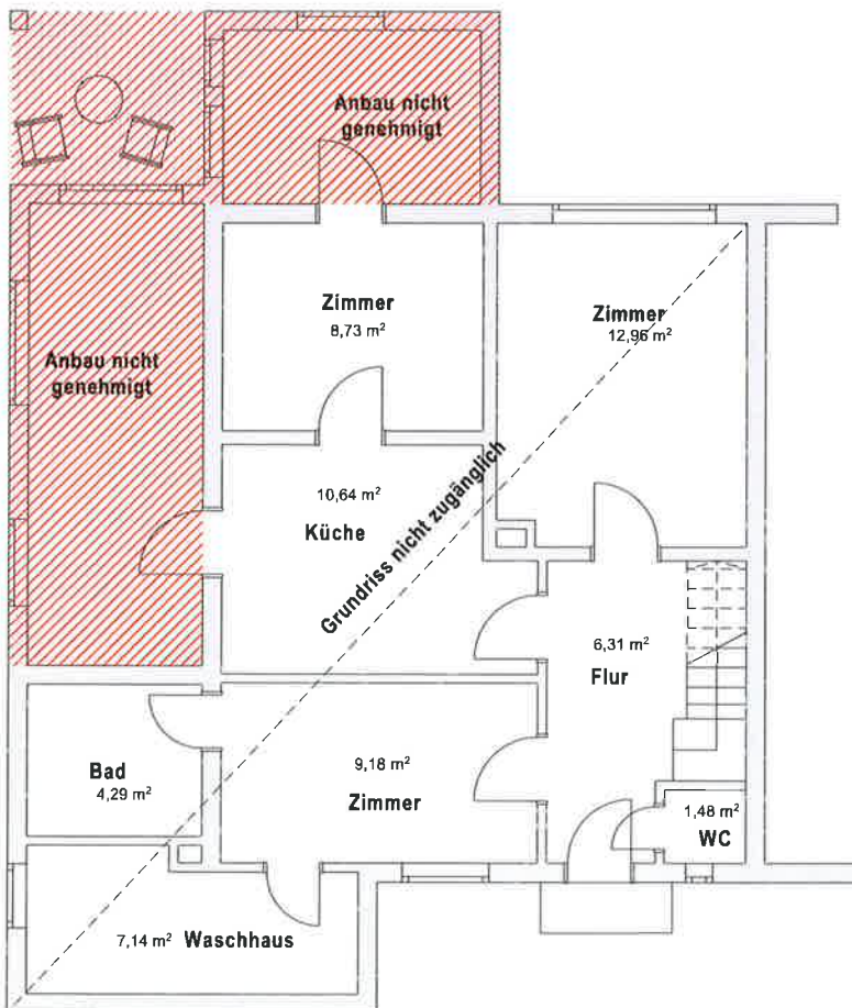
Erdgeschoss
